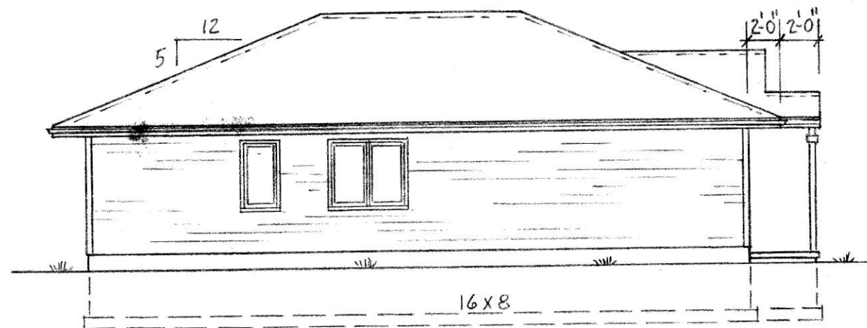
LEFT ELEV. 1/8" = 1'-0"
