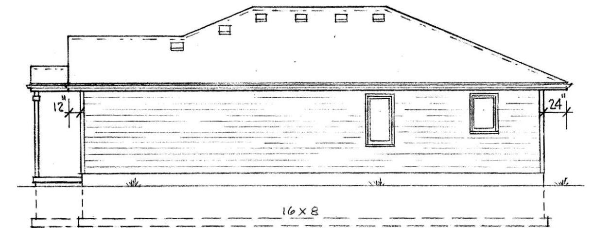
RIGHT ELEV.
